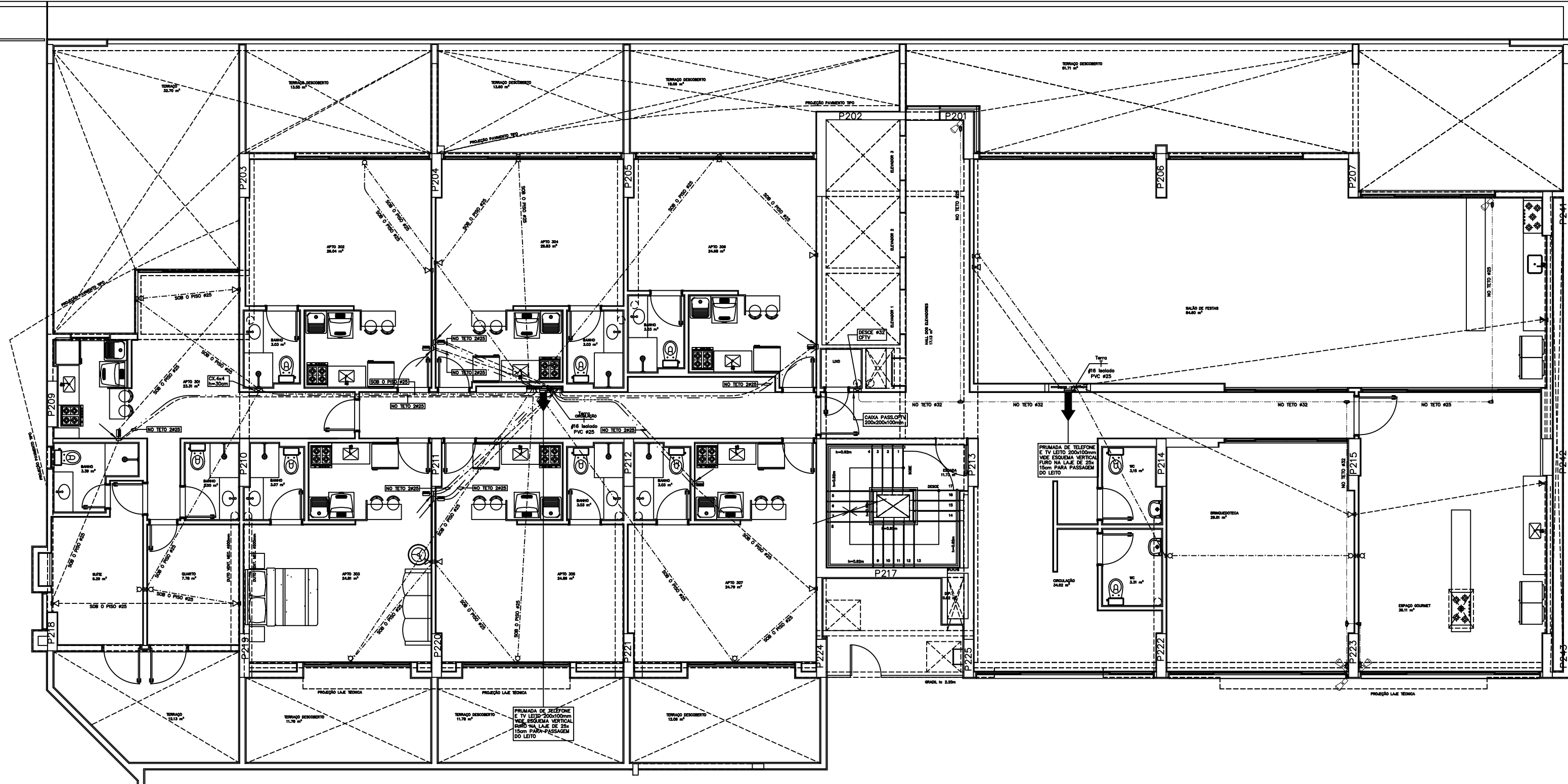
PLANTA BAIXA 3º PAVIMENTO – BLOCO "B" RESIDENCIAL ESCALA 1:50
