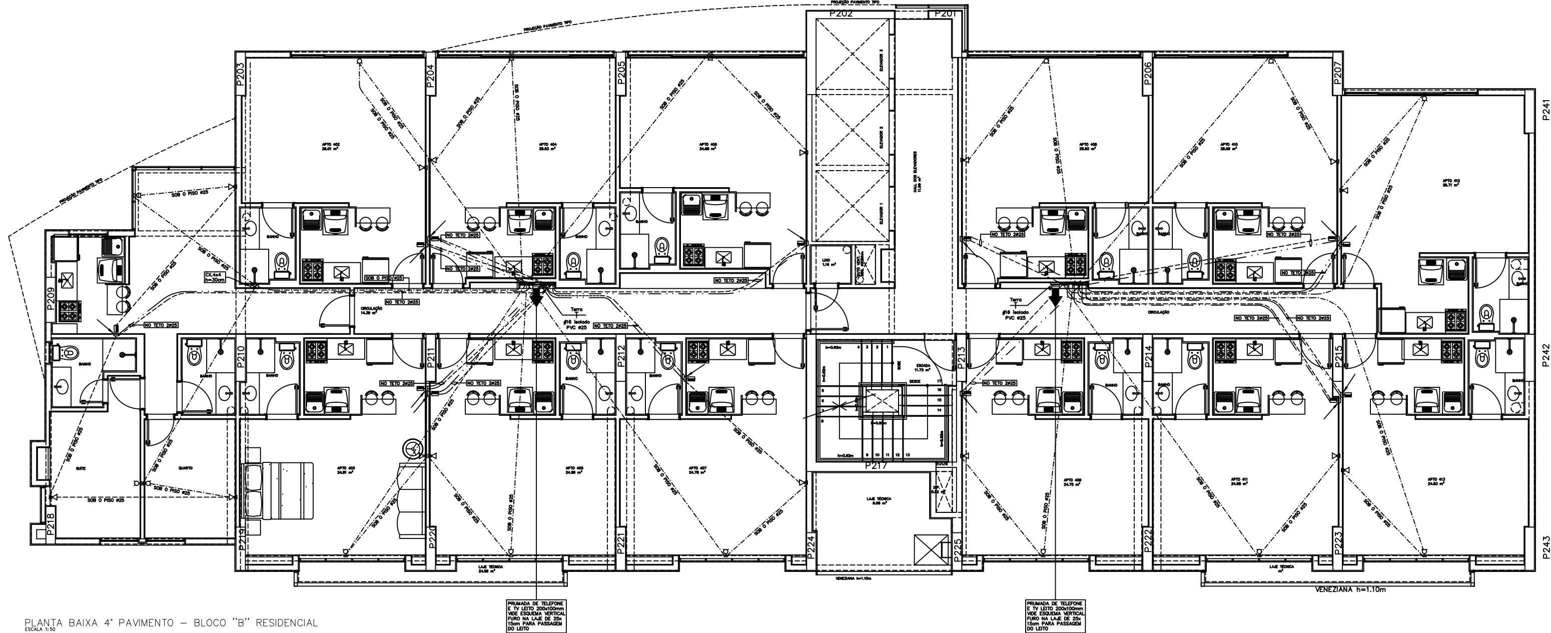
PLANTA BAIXA 4º PAVIMENTO – BLOCO "B" RESIDENCIAL ESCALA 1:50
